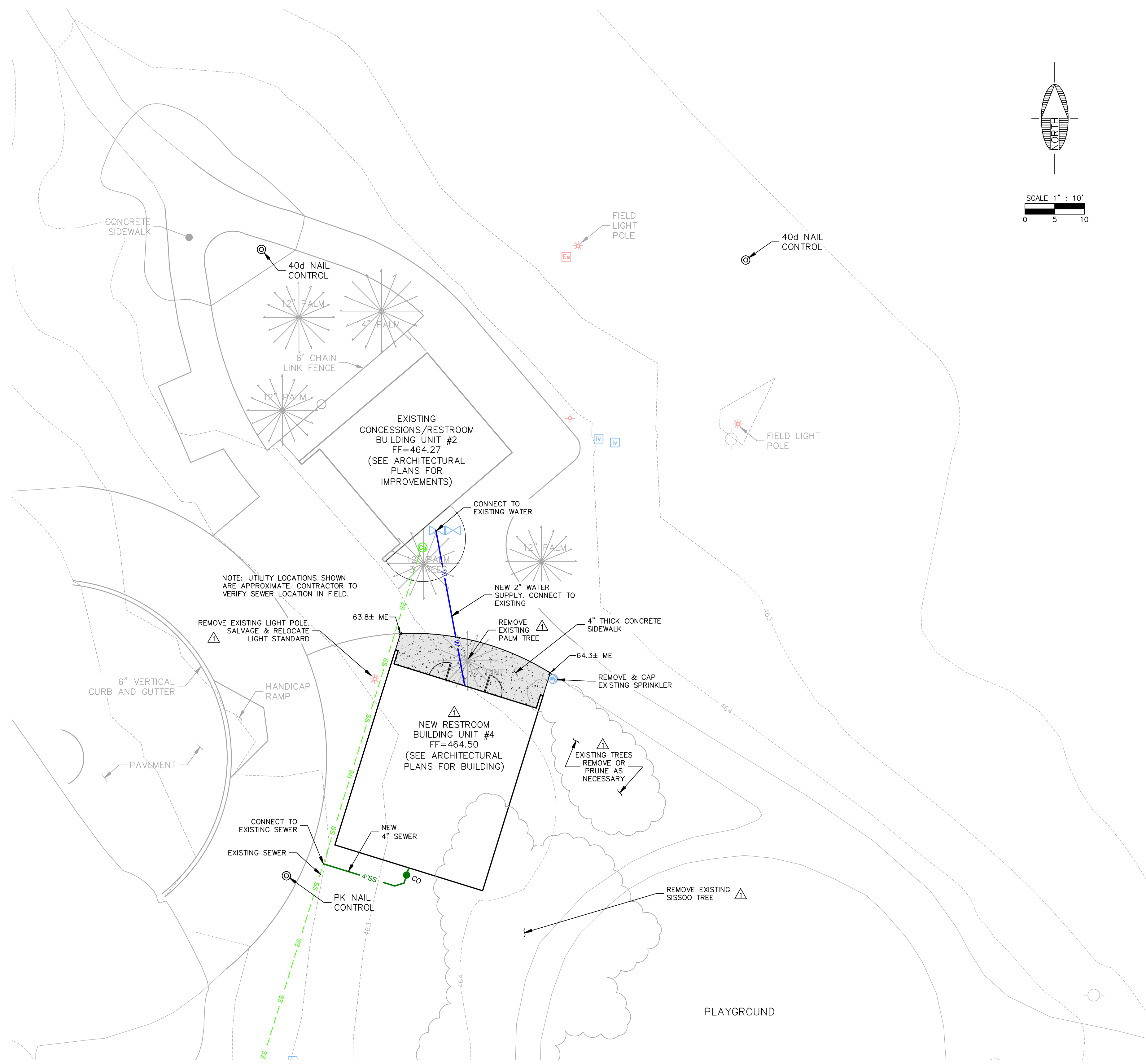
SITE PLAN 1"=10'
